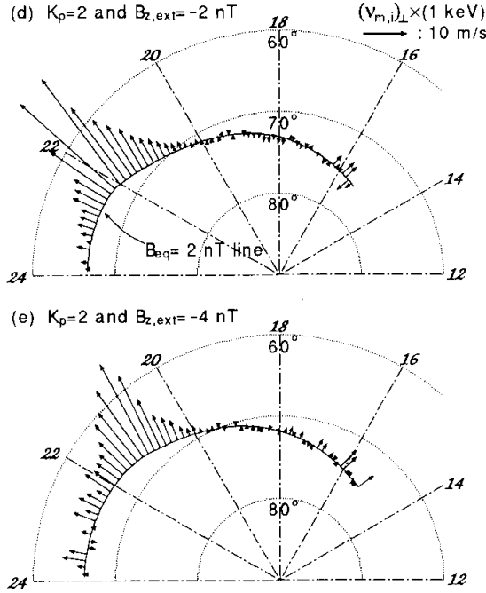
Fig. 10 (continued). (d) K_p=2 and B_{z,ext}=-2 nT, and (e) K_p=2 and B_{z,ext}=-4 nT.
