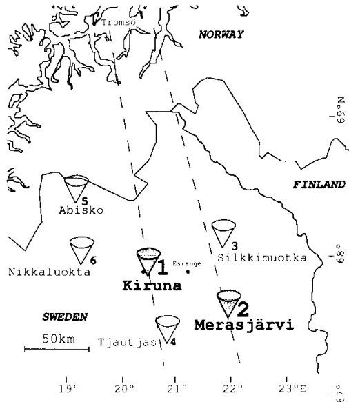
Fig. 5. ALIS observation site map.
